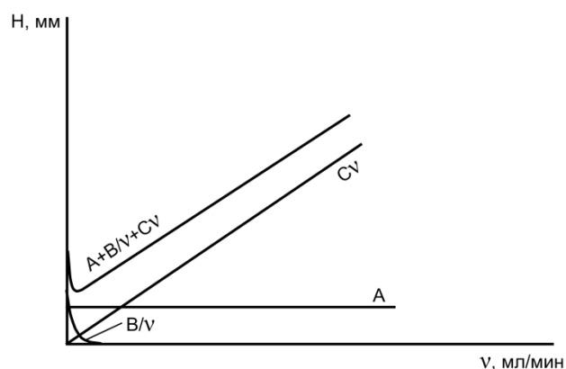
Рис. 7. Зависимость ВЭТТ от скорости потока элюента. Вклад в размывание пика разных факторов.
