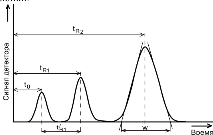
Рис. 5. Хроматограмма смеси двух веществ, полученная элюентным методом.
