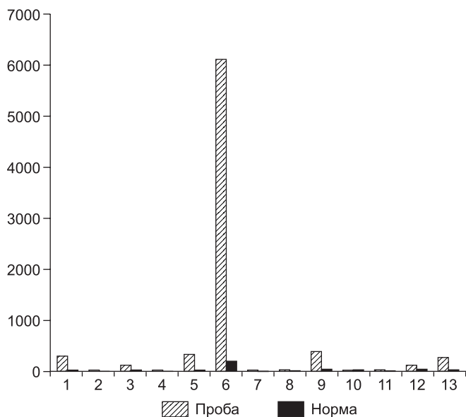
Рис. 2. Реконструкции состава МО по микробным маркерам в моче ребенка 11 лет, больного пиелонефритом.
