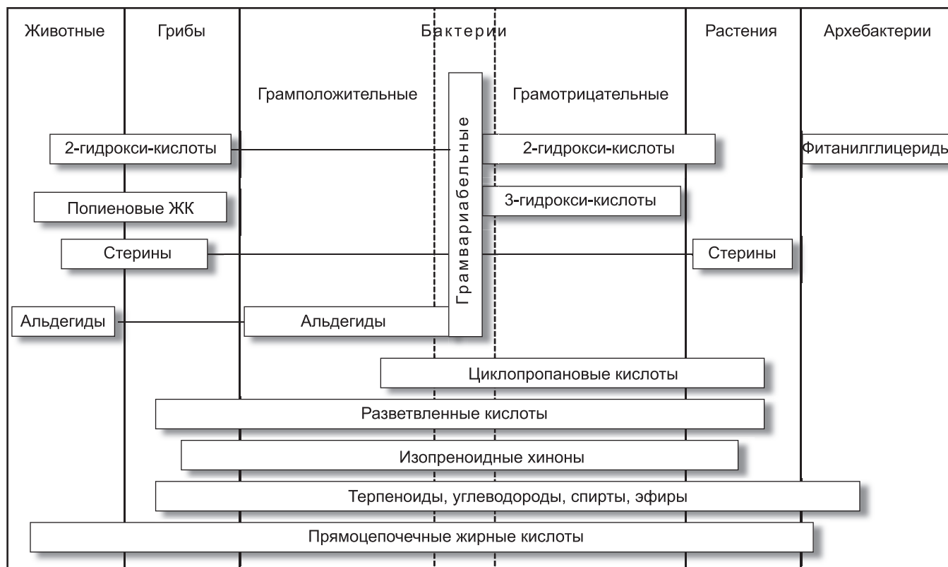
Рис. 1. Многообразие липидных компонентов клеток. Животные, растения и МО разных царств и родов имеют как общие, так и отличительные структурные компоненты липидов.
