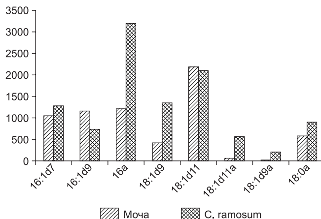
Рис. 3. Сопоставление распределения ключевых маркеров клостридий C. ramosum с их соотношением в моче ребенка. Приведена общепринятая аббревиатура ЖК и альдегидов (см. таблицу). Последние отмечены буквой а в конце символа.
